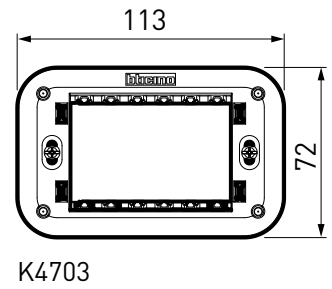
4 MODÜL KAİDE
