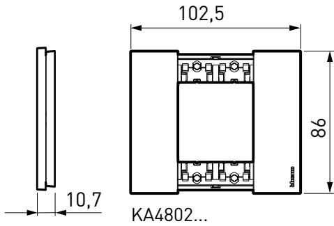
2 MODÜL ÇERÇEVE
