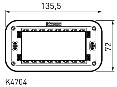
6 MODÜL KAİDE
