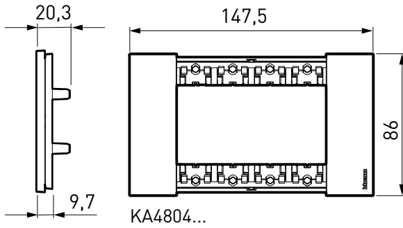
4 MODÜL ÇERÇEVE
