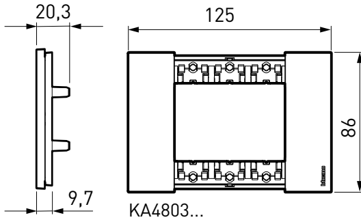
3 MODÜL ÇERÇEVE
