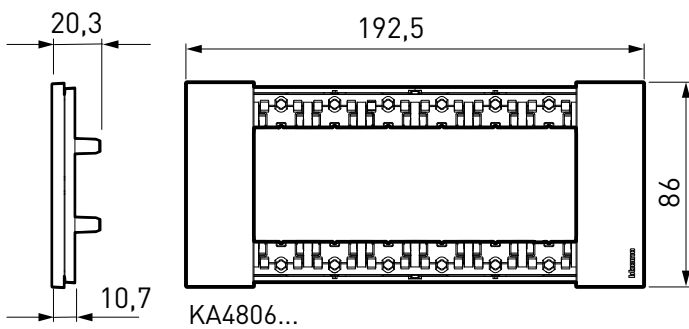
6 MODÜL ÇERÇEVE
